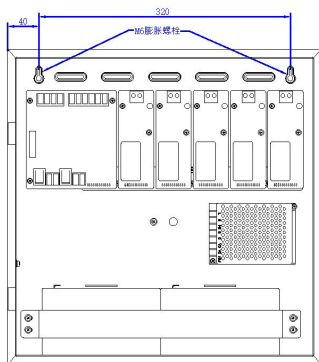
图 2-7 安装结构
