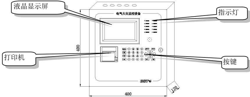
图 2-1 外观示意图
